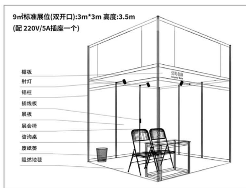
标准展位为 9 平方米 (3 米 * 3 米), 基本设施配备如上 (单位: mm)
